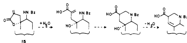
Scheme VI
